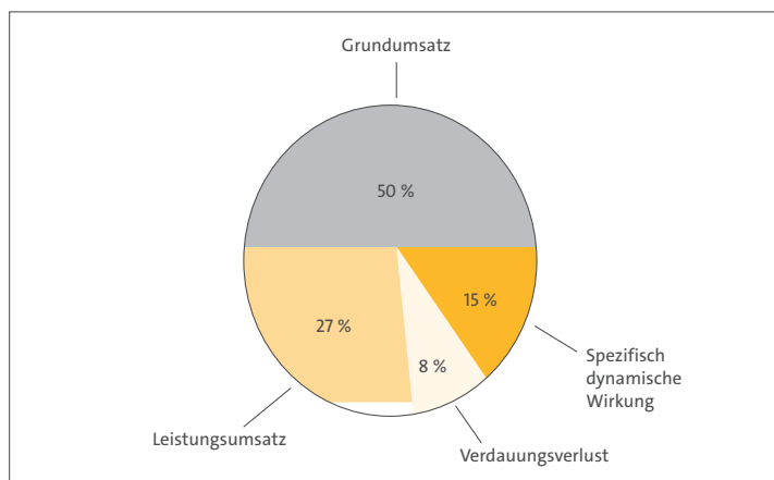
Abb. 6 Zusammensetzung des Energiebedarfs bei normaler körperlicher Belastung (in Anlehnung an WEINECK 2004, S. 624)
